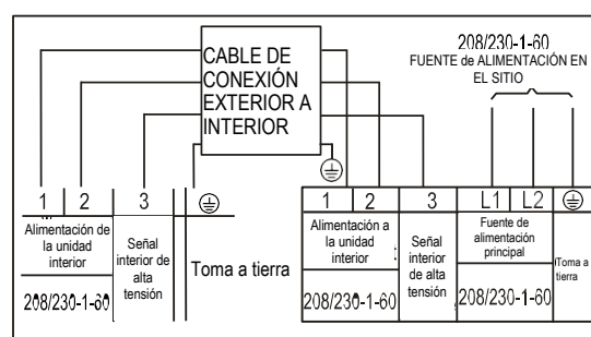
Diagrama de conexión (208/230 V)
