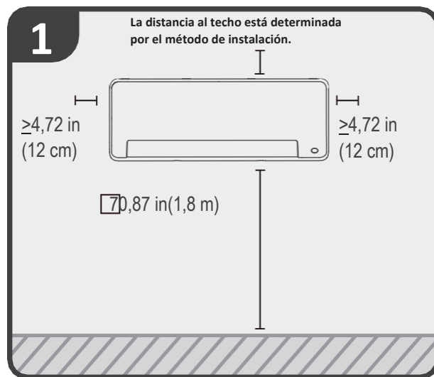
Elegir el lugar de la instalación
