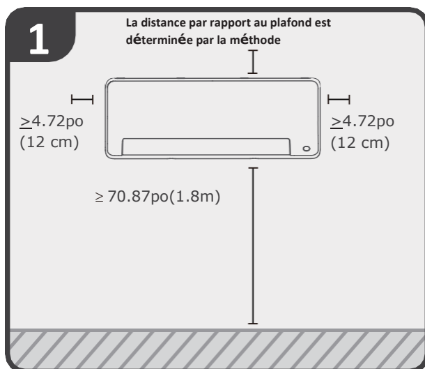
Choisir le lieu de l'installation
