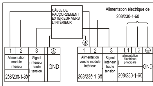
Schéma de connexion (208/ 230V)
