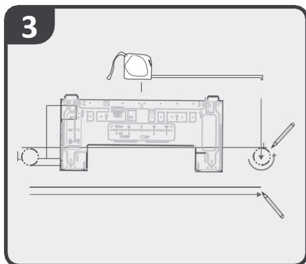
Déterminez la position du trou sur le mur
