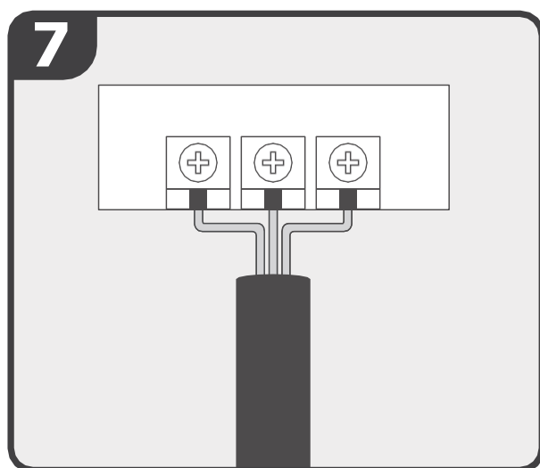
Raccordement du câblage
