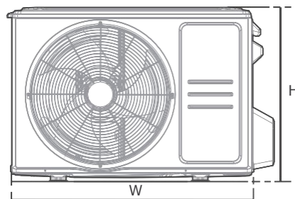
Vue avant
