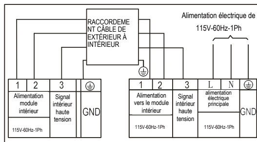
Schéma de connexion (115V)
