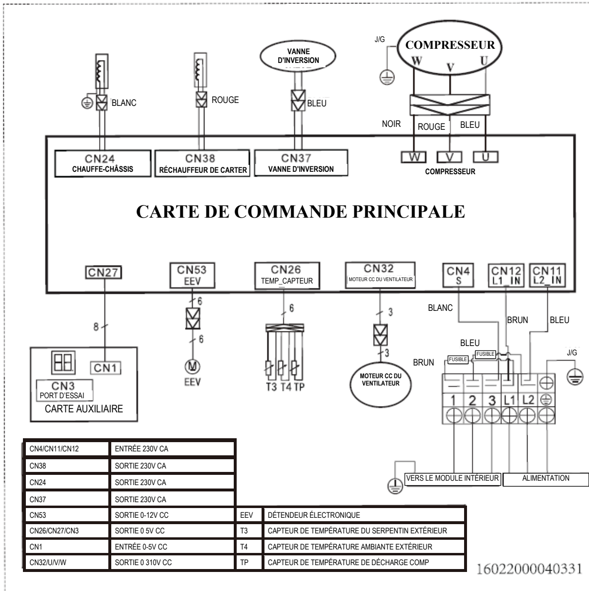
Schéma de câblage du module extérieur : 16022000040331
