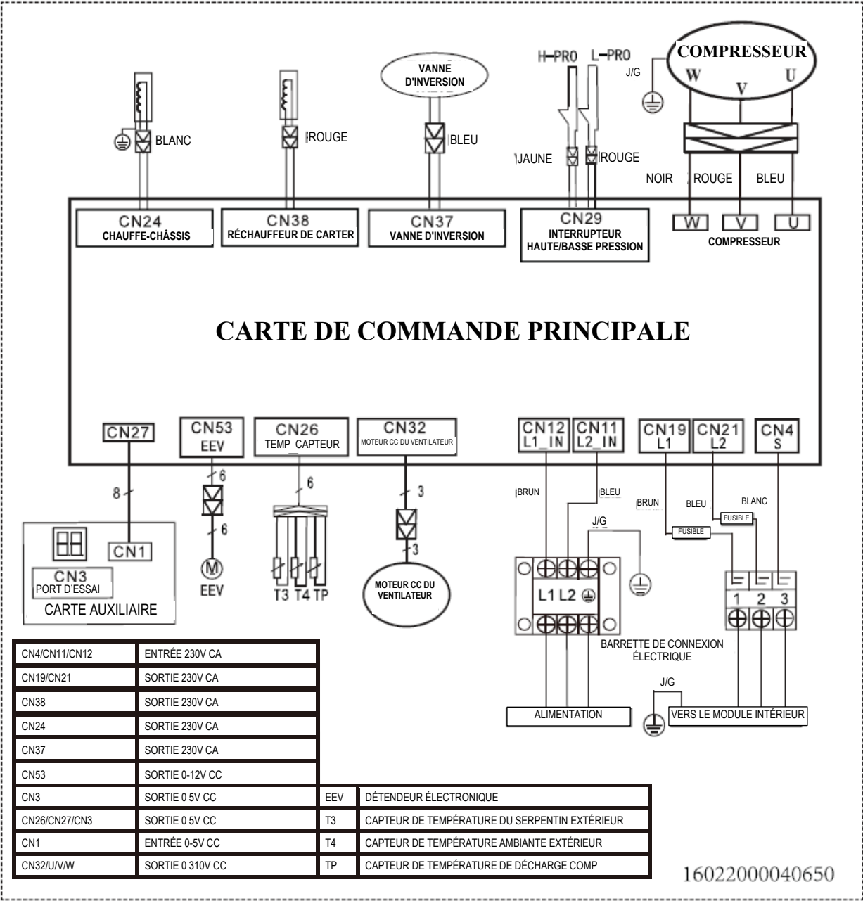
Schéma de câblage du module extérieur : 16022000040650
