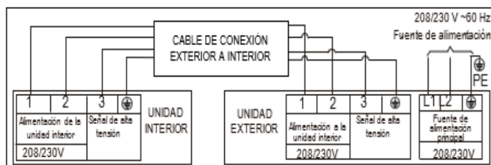
Diagrama de conexión (9K/12K/16K)
