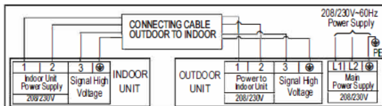
Schéma de connexion (9K/1 2 K/16K)
