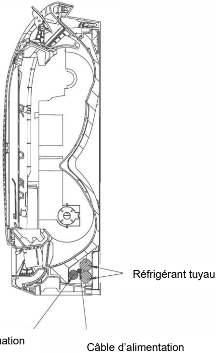
Câble d'alimentation
