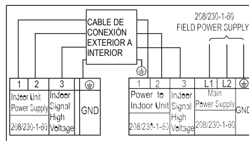
Diagrama de conexión (208/230 V)
