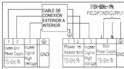
Diagrama de conexión (115 V)
