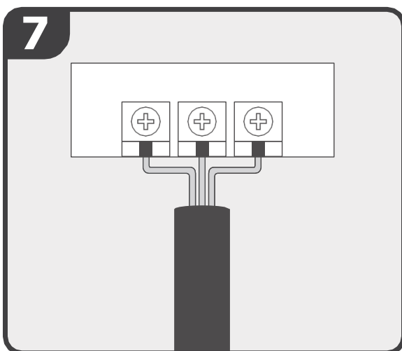
Conectar el cableado
