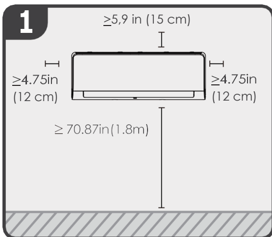
Elegir el lugar de la instalación
