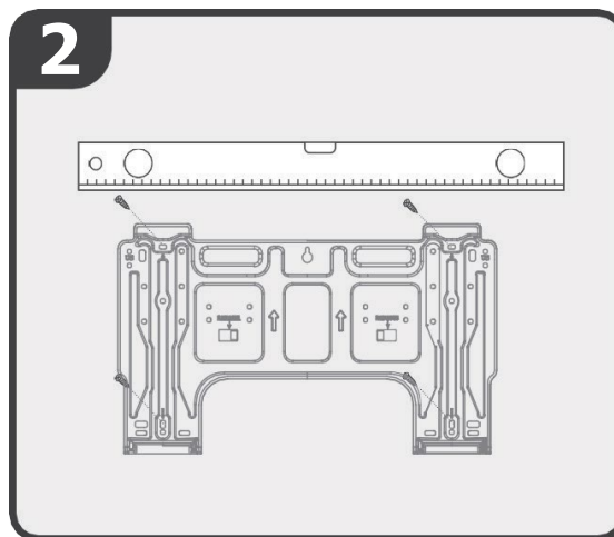
Fijar la placa de montaje
