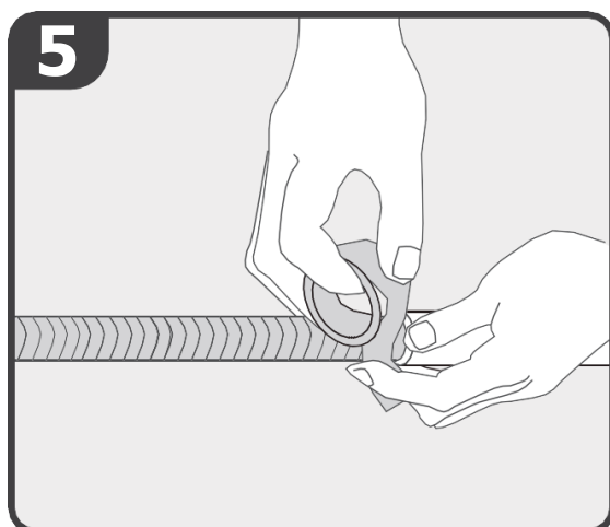
Preparar la manguera de desagüe
